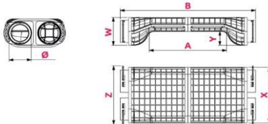
Dimenzije (mm)
