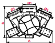
Dimenzije (mm)
