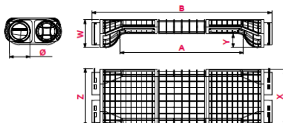
Dimenzije (mm)
