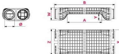
Dimenzije (mm)
