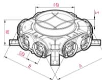
Dimenzije (mm)
