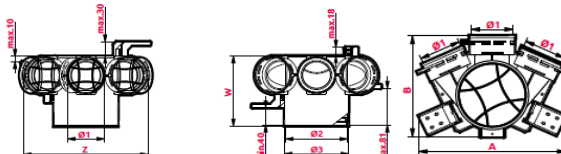
Dimenzije (mm)
