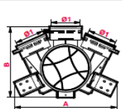
Dimenzije (mm)
