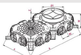
Dimenzije (mm)
